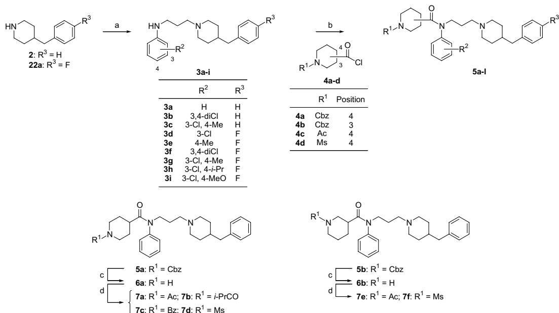
Scheme 1. Reagents: (a) acrolein, cat. DBU, THF, then R 2 -PhNH 2 , NaBH(OAc) 3 ; (b) 4a–d , Et 3 N, DCM; (c) H 2 , Pd/C, MeOH; (d) R 1 -Cl, Et 3 N, THF.
