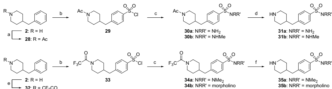
Scheme 6. Reagents: (a) \text{Ac}_2\text{O} ; (b) \text{ClSO}_3\text{H} , DCM; (c) \text{HNRR}' , (\text{Et}_3\text{N}) , THF; (d) concd \text{HCl} ; (e) TFAA; (f) \text{K}_2\text{CO}_3 , \text{H}_2\text{O} , MeOH.
