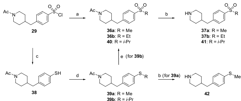
Scheme 7. Reagents: (a) \text{Na}_2\text{SO}_3 , \text{NaHCO}_3 , \text{H}_2\text{O} , then \text{ClCH}_2\text{CO}_2\text{H} or \text{CH}_3\text{CH}(\text{Br})\text{CO}_2\text{H} , aq \text{NaOH} ; (b) concd \text{HCl} , then aq \text{NaOH} ; (c) \text{Zn} , \text{H}_2\text{SO}_4 ; (d) \text{RI} , \text{K}_2\text{CO}_3 , DMF; (e) m\text{CPBA} , DCM.
