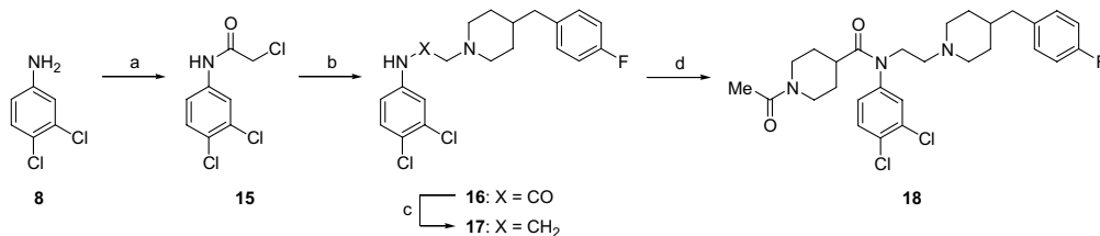
Scheme 3. Reagents: (a) (\text{ClCH}_2\text{CO})_2\text{O} , \text{THF} ; (b) 22a , \text{K}_2\text{CO}_3 , \text{DMF} ; (c) \text{BH}_3 \cdot \text{Me}_2\text{S} , \text{THF} ; (d) 4c , \text{Et}_3\text{N} , \text{DCM} .
