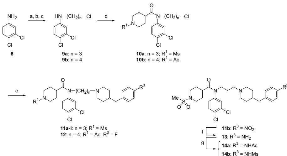
Scheme 2. Reagents: (a) \text{HCO}_2\text{Ac} ; (b) \text{Br}(\text{CH}_2)_n\text{Cl} , \text{Cs}_2\text{CO}_3 , acetone; (c) concd \text{HCl} , i\text{-PrOH} ; (d) 4d or 4c , \text{Et}_3\text{N} , \text{DCM} ; (e) 4-( R^3 -benzyl)piperidine, \text{KI} , \text{K}_2\text{CO}_3 , \text{MeCN} ; (f) \text{SnCl}_2 \cdot 2\text{H}_2\text{O} , \text{EtOH} ; (g) \text{AcCl} or \text{MsCl} , \text{Et}_3\text{N} , \text{THF} .
