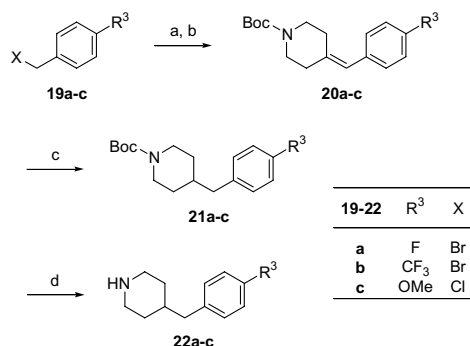
Scheme 4. Reagents: (a) (\text{EtO})_3\text{P} ; (b) 1-Boc-4-piperidone, \text{NaH} , \text{THF} ; (c) \text{H}_2 , \text{Pd/C} , \text{MeOH} ; (d) \text{HCl} , \text{EtOAc} .
